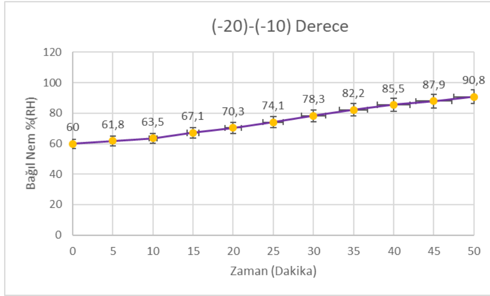
Şekil 7. Kaskad Soğuk Depolarda Ultrasonik Nemlendirme ile (-20°)- (-10°)sıcaklık aralığında bağıl nem grafiği
