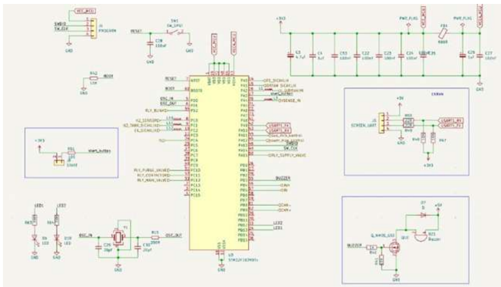
Şekil 10. Mikrodenetleyici devresi
