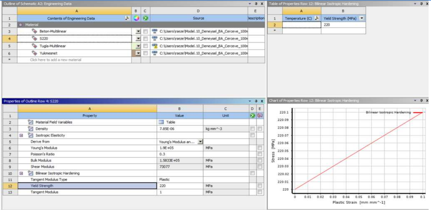
Şekil 3.2 S220 Donatısı için Bilinear Isotropic Hardening Modeli
