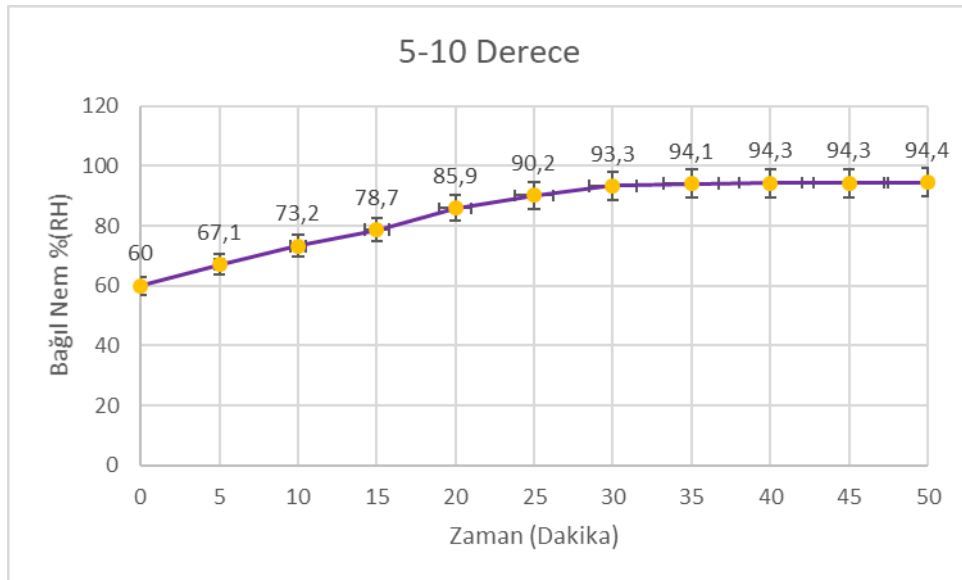
Şekil 5. Kaskad Soğuk Depolarda Ultrasonik Nemlendirme ile 5°-10° sıcaklık aralığında bağıl nem grafiği
