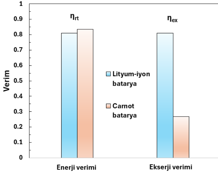
Şekil 7. Enerji ve ekserji verimleri
