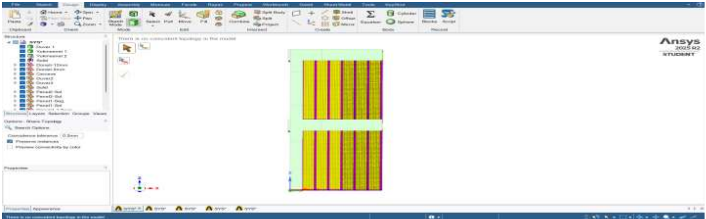
Şekil 4.7 B Tipi Numune Solid Modelinin Oluşturulmuş Hali
