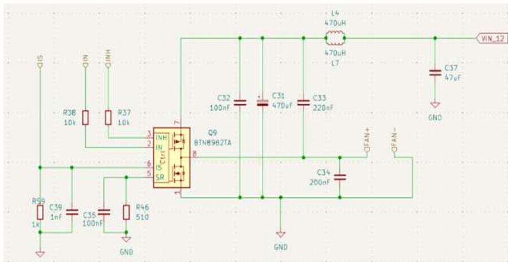
Şekil 11. Fan kontrol devresi
