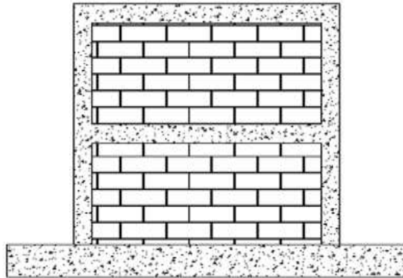
Şekil. 2.1 Referans Numune (RN) Modeli
