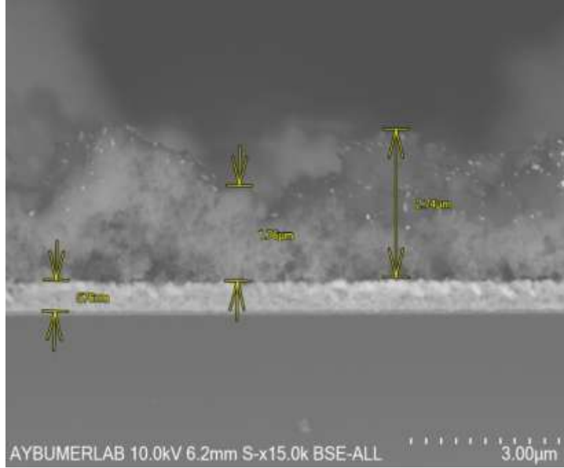
Şekil 1. FTO üzerinde \text{TiO}_2 -PDA-UiO66-Au kompozit elektrodunun kesit SEM görüntüsü
