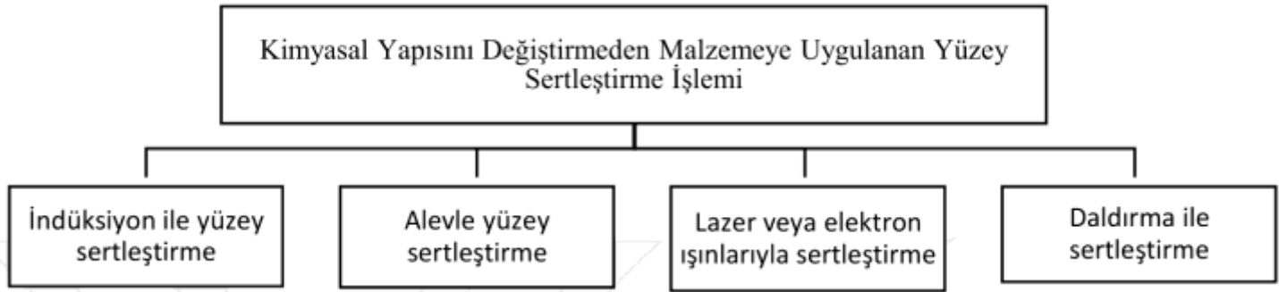
Şekil 1. Kimyasal Yapı Değişmeden Yapılan Sertleştirme İşlemi (Demirtaş, 2024)
