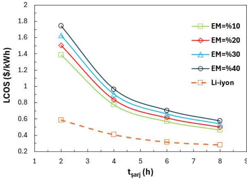
Şekil 5. Seviyelendirilmiş enerji depolama maliyetinin (LCOS) ek maliyet oranına (EM) ve şarj süresine bağlı değişimi (300 kW kapasite)
