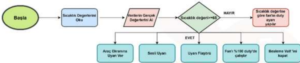
Şekil 7. Termal Yönetim Algoritması
