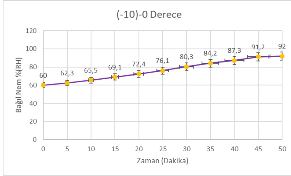
Şekil 6. Kaskad Soğuk Depolarda Ultrasonik Nemlendirme ile (-10°)-0° sıcaklık aralığında bağıl nem grafiği
