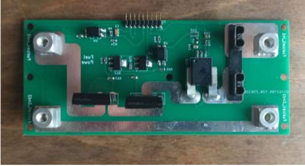
Şekil 14. Güç Kartı
