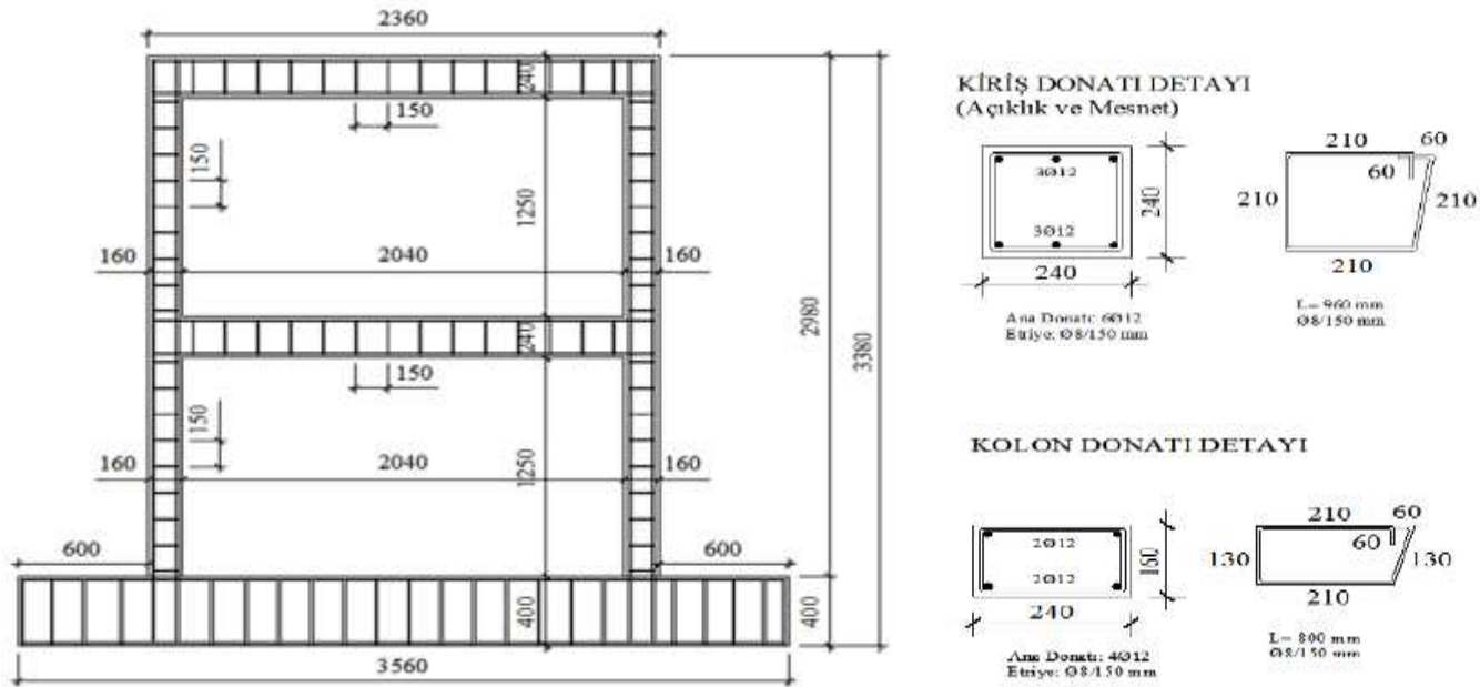
Şekil.2.4 Betonarme Çerçevenin Donatı Düzeni
