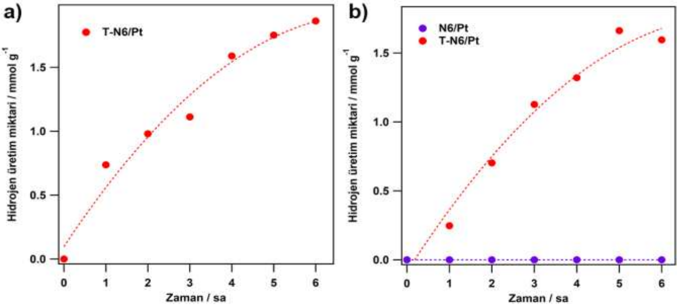
Şekil 6. N6, boyar maddesi ve TiO 2 fotokatalizörlerinin a) sentezli ve b) ortamda Pt yardımcı katalizörünün varlığında elde edilen 6 saatlik fotokatalitik hidrojen üretim aktiviteleri.
