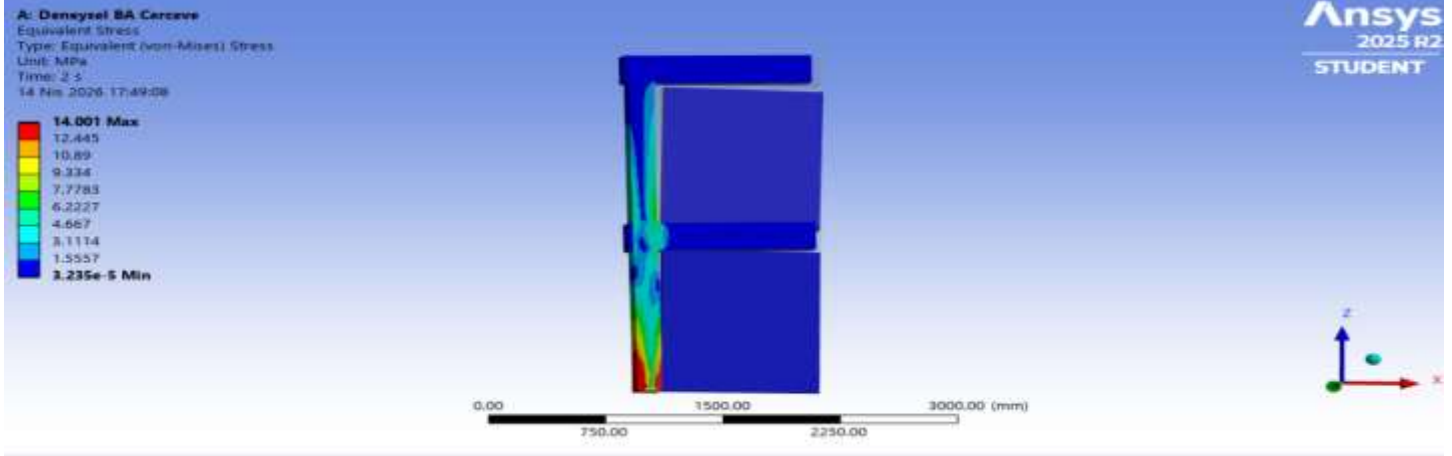
Şekil 6.1 Referans Numune Eşdeğer Von-Mises Beton Gerilmesi
