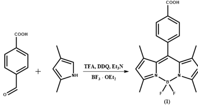
Şekil 1. 4'-difloro-8-(p-karboksifenil)-1,3,5,7-tetrametil-4-bora-3a,4a-diaza-s-indasen (N6) sentezi.
