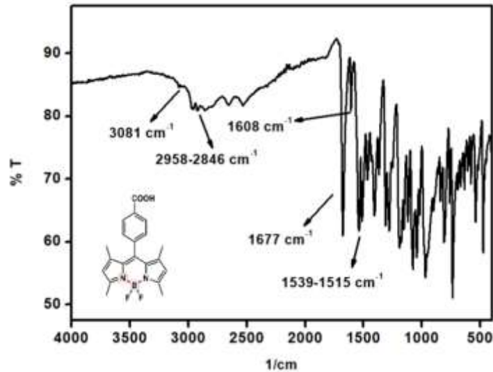
Şekil 3. 4'-difloro-8-(p-karboksifenil)-1,3,5,7-tetrametil-4-bora-3a,4a-diaza-s-indasen (N6) bileşiğinin FTIR spektrumu.
