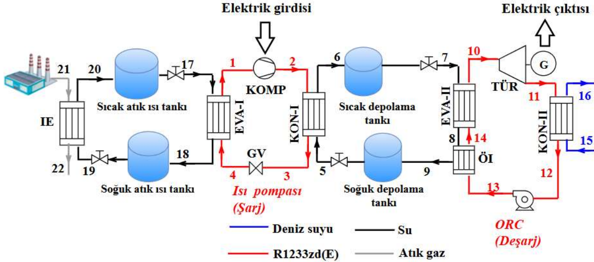
Şekil 2. Carnot batarya sistemi
