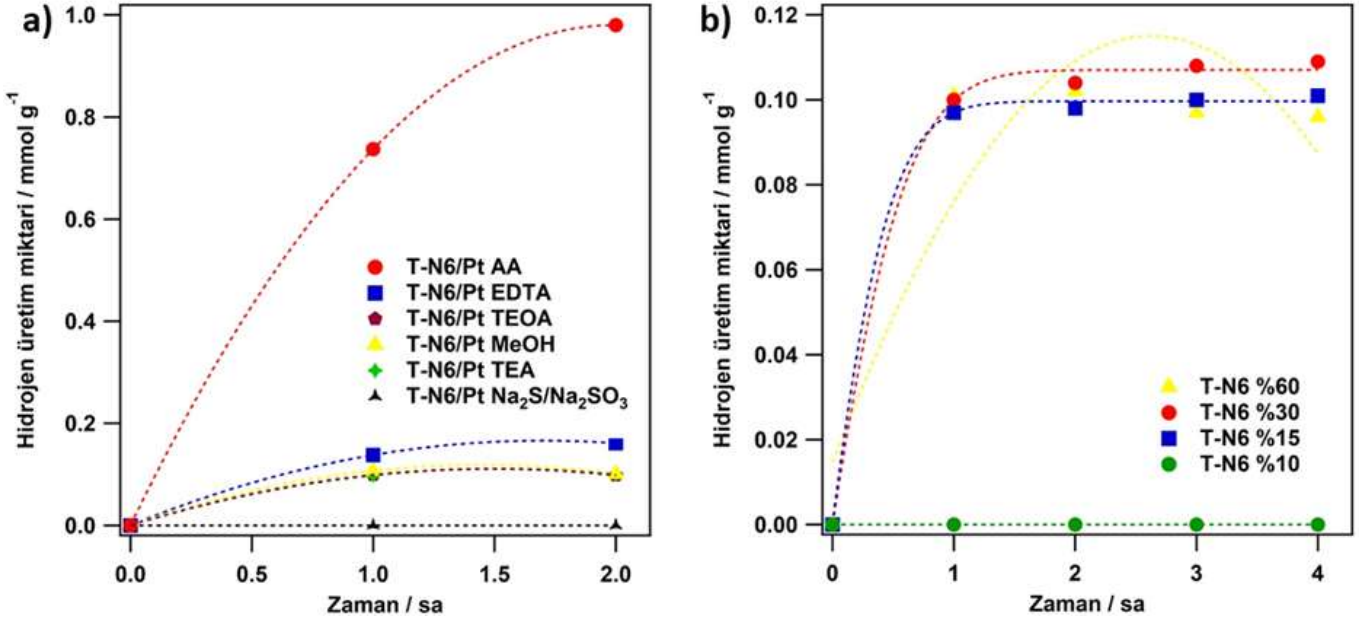
Şekil 5. T-N6 fotokatalizörünün fotokatalitik hidrojen üretiminde a) Farklı elektron verici etkisi ve b) İkili ve üçlü yapıları.
