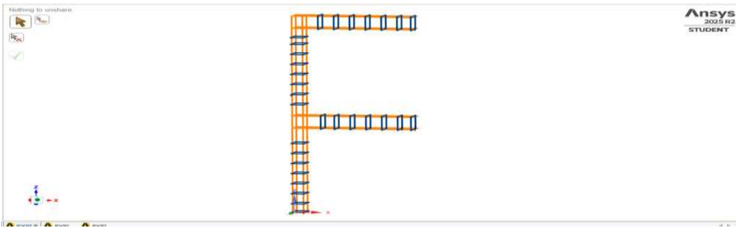
Şekil 4.3 Referans Numune Donatı Düzenin Üç Boyutlu Hali
