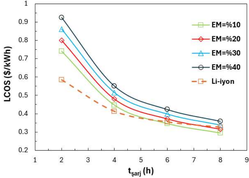
Şekil 3. Seviyelendirilmiş enerji depolama maliyetinin (LCOS) ek maliyet oranına (EM) ve şarj süresine bağlı değişimi (1800 kW kapasite)
