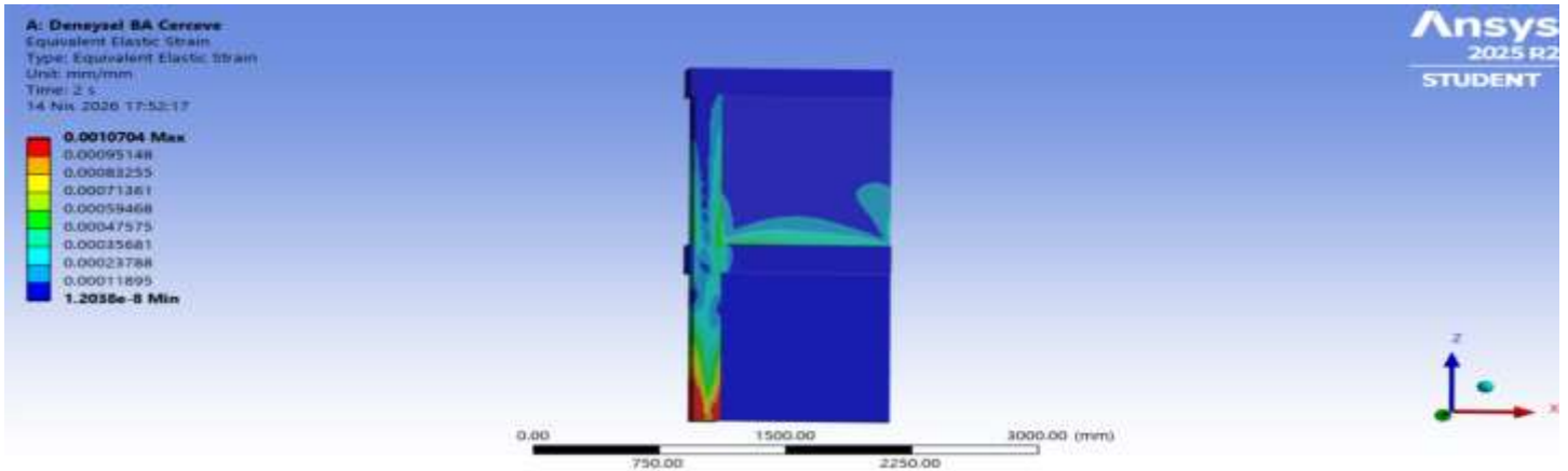
Şekil 6.3 Referans Numune x Yönünde Eşdeğer Elastik Şekil Değiştirmesi
