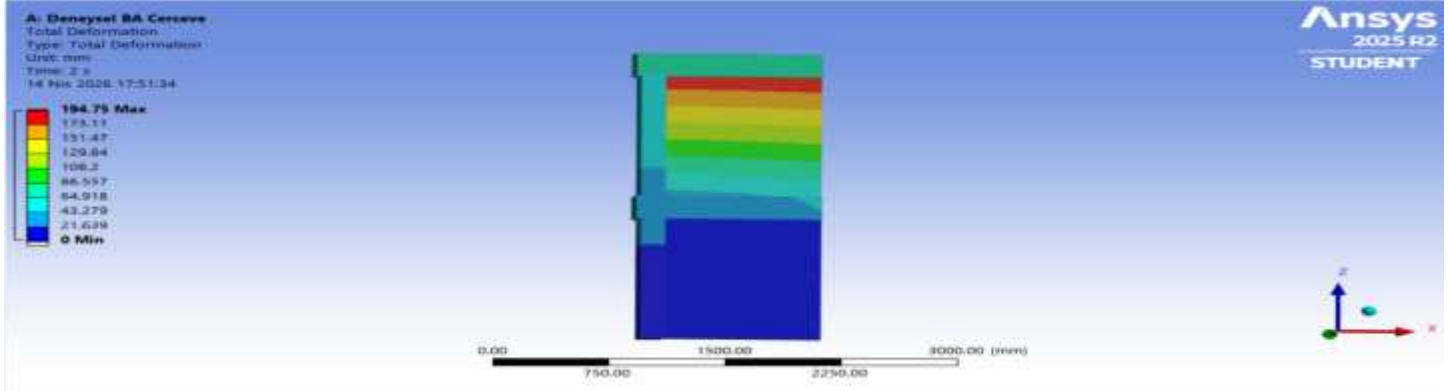
Şekil 6.4 Referans Numune Toplam Deformasyonu
