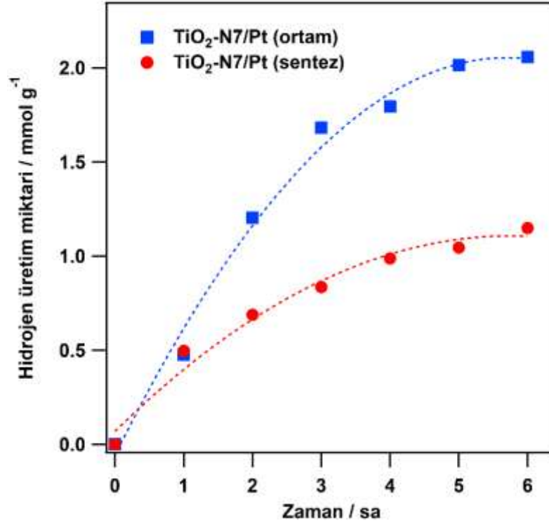
Şekil 3. Sentezli ve ortam koşullarında hazırlanan N7 ile hassaslaştırılmış TiO 2 /Pt fotokatalizörlerinin görünür ışık altında zamana bağlı hidrojen üretim miktarlarının karşılaştırılması.
