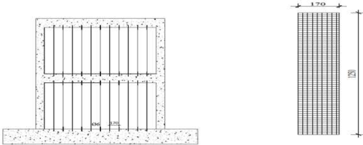
Şekil 2.3 Dikdörtgen Pannelle (B Tipi ) Güçlendirilmiş Dolgulu Numune Modeli
