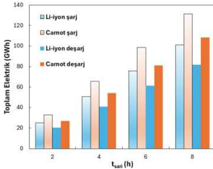
Şekil 4. 25 yıllık sistem ömrü boyunca depolanan ve şarj edilen toplam elektrik miktarı (1800 kW kapasite)
