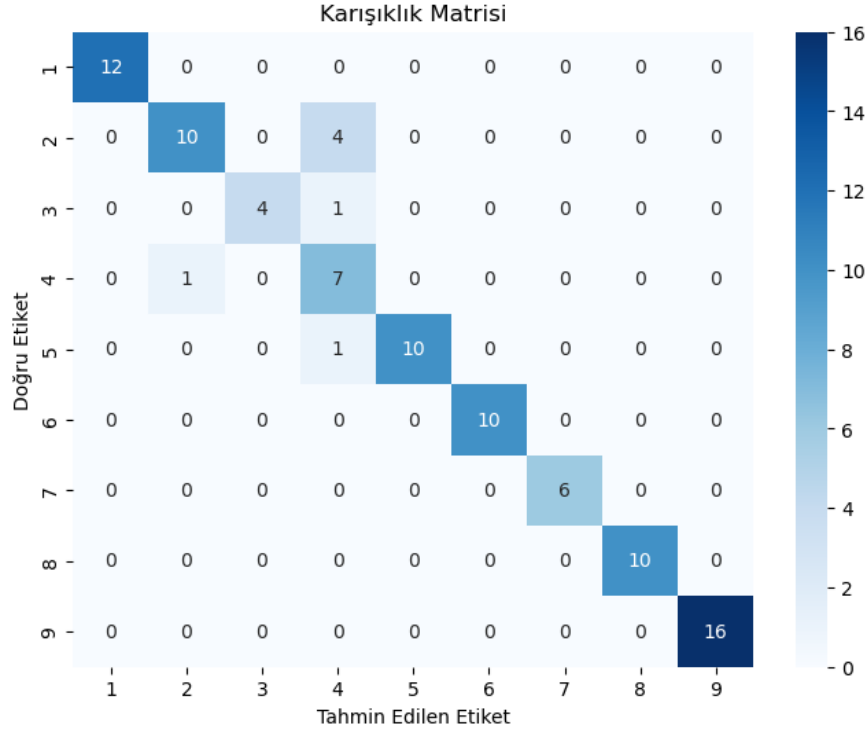
Şekil 21. SVM Modeli Karmaşıklık Matrisi
