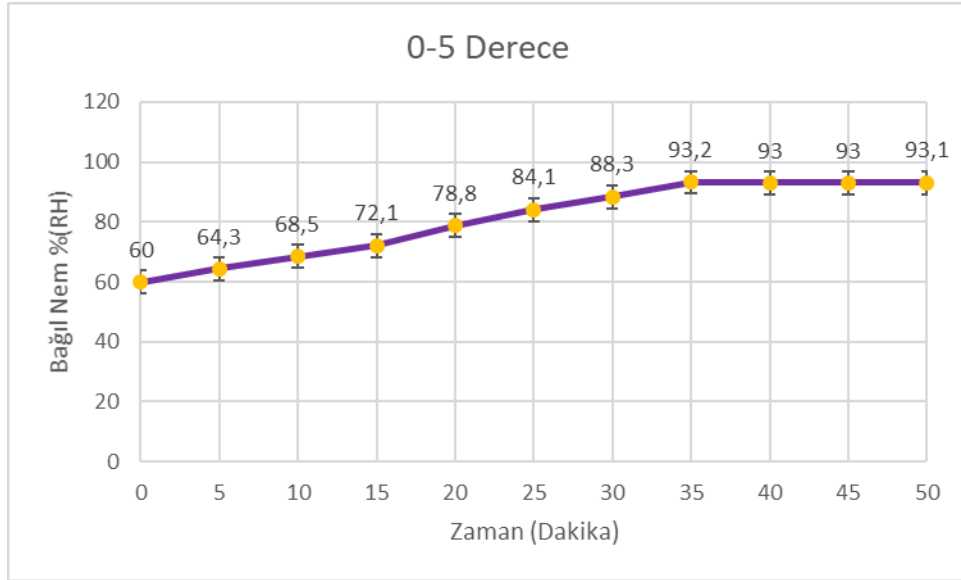
Şekil 4. Kaskad Soğuk Depolarda Ultrasonik Nemlendirme ile 0°-5° sıcaklık aralığında bağıl nem grafiği
