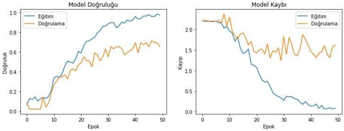
Şekil 19. CNN Modeli Doğruluk ve Kayıp Eğrileri
