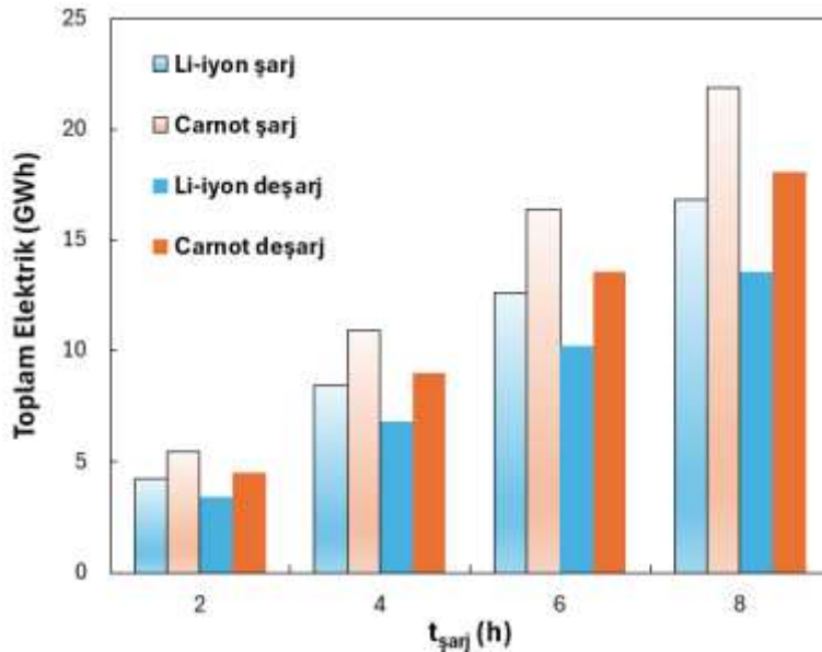
Şekil 6. 25 yıllık sistem ömrü boyunca depolanan ve şarj edilen toplam elektrik miktarı (300 kW kapasite)
