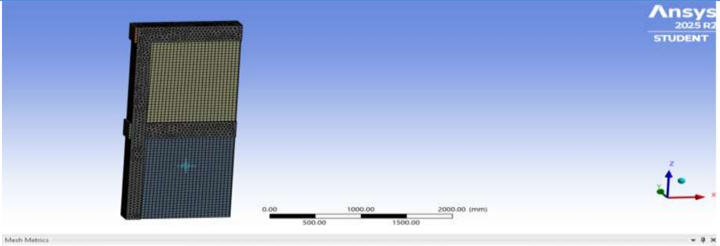
Şekil 5.1 Referans Numune Sonlu Eleman Ağı
