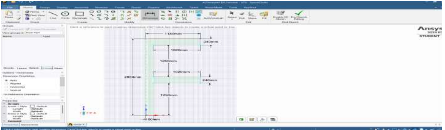
Şekil 4.1 Referans Numune Solid Modelinin xz Düzlemindeki Boyutları
