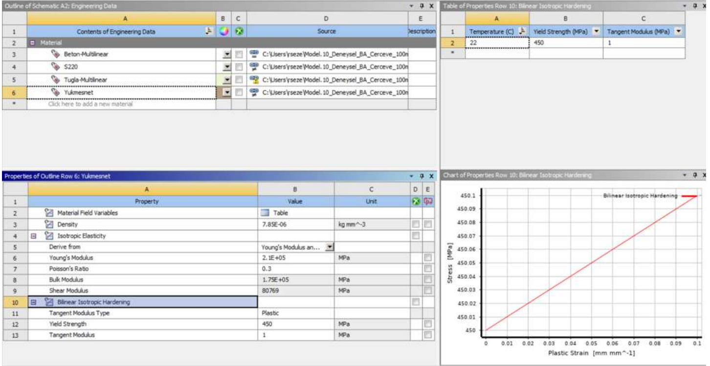
Şekil 3.4 S450 Yük Mesnet Levhası için Bilinear Isotropic Hardening Çelik Modeli
