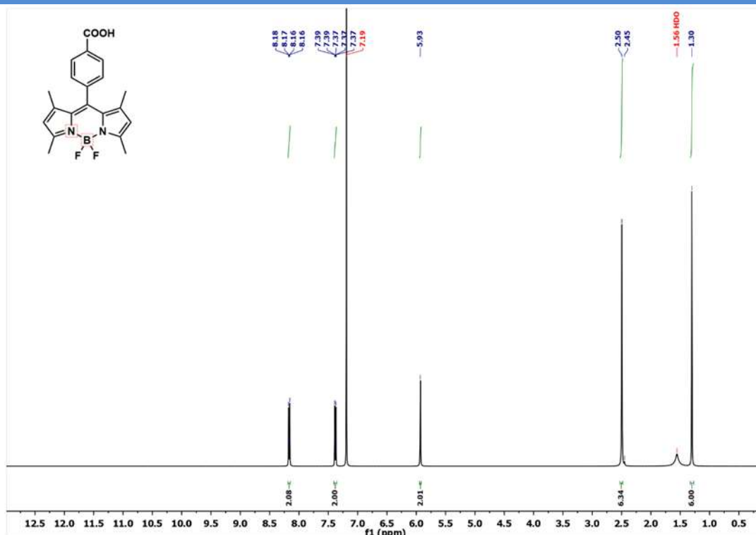
Şekil 4. 4'-difloro-8-(p-karboksifenil)-1,3,5,7-tetrametil-4-bora-3a,4a-diaza-s-indasen (N6) bileşiğinin d-CDCl 3 içerisinde alınan 1 H-NMR spektrumu.
