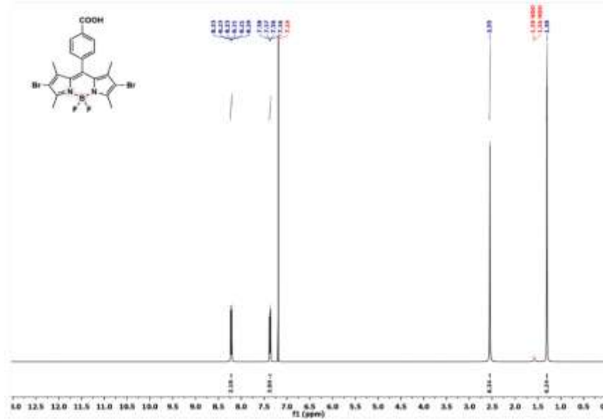
Şekil 2. 4,4'-difluoro-8-( p -karboksifenil)-2,6-dibromo-1,3,5,7-tetrametil-4-bora-3a,4a-diaza-s-indasen (N7) bileşiğinin d-CDCl 3 içerisinde alınan 1 H-NMR spektrumu.
