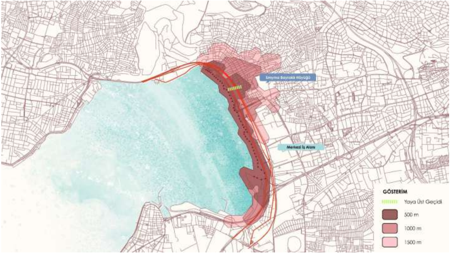
Şekil 5: Çalışma alanına ilişkin 500m.,1000m. ve 1500m. servis alanı analizi
