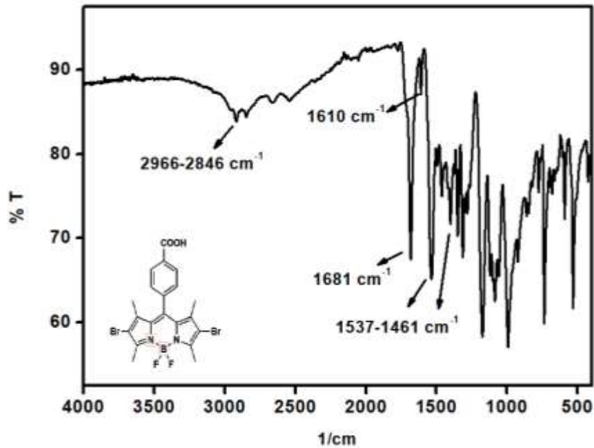
Şekil 1. 4,4'-difloro-8-(p-karboxifenil)-2,6-dibromo-1,3,5,7-tetrametil-4-bora-3a,4a-diaza-s-indasen (N7) bileşiğinin FTIR spektrumu.
