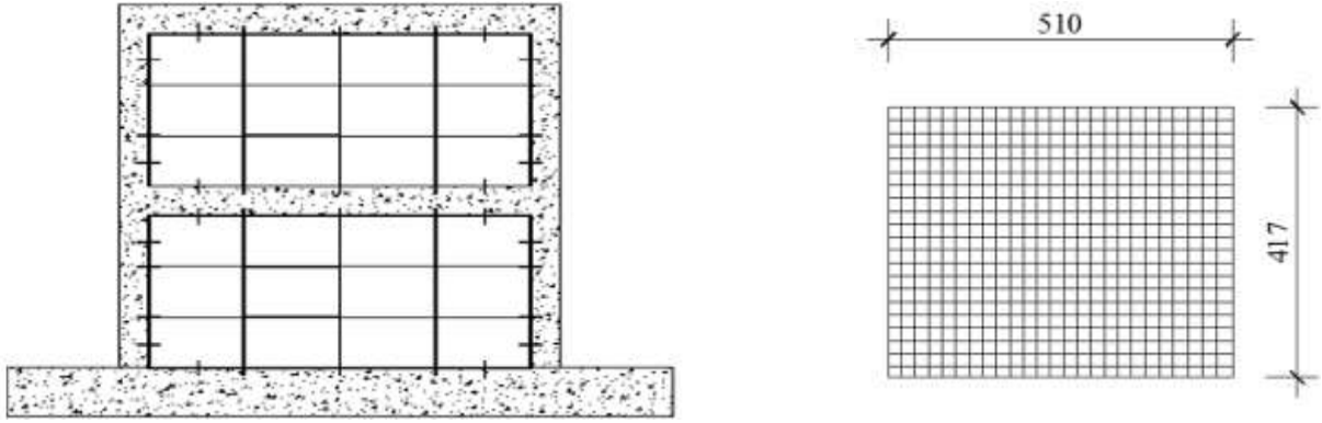
Şekil 2.2 Kare Pannelle (A Tipi) Güçlendirilmiş Dolgulu Numune Modeli
