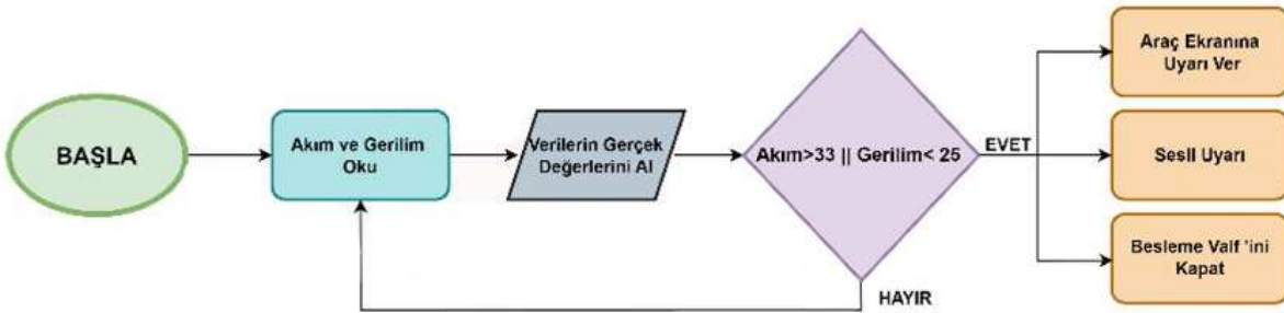
Şekil 8. Akım ve Gerilim Yönetim Algoritması
