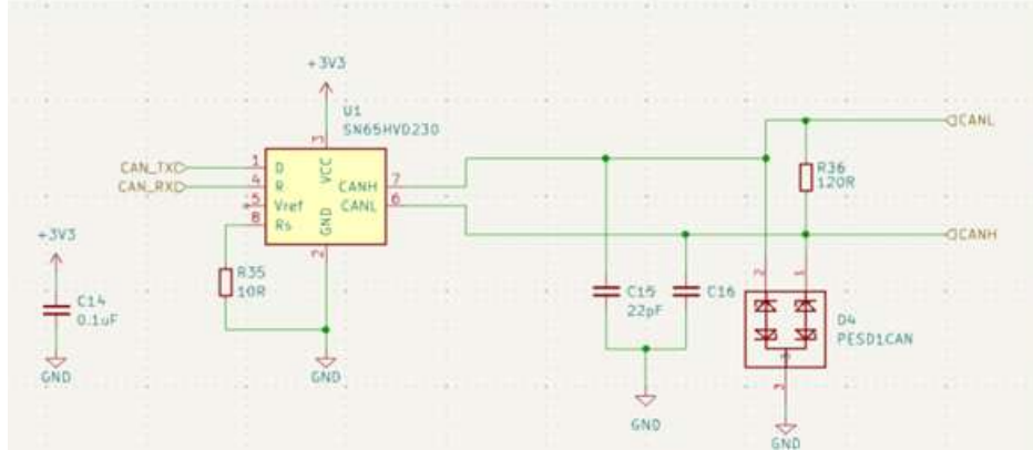
Şekil 12. CAN-BUS devresi
