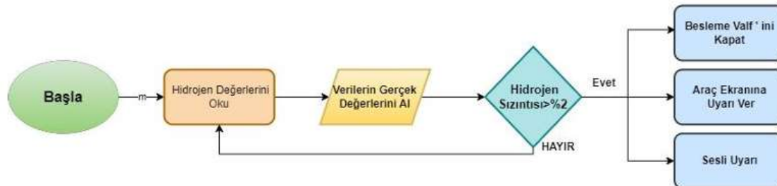
Şekil 9. Hidrojen Sızıntı Algoritması
