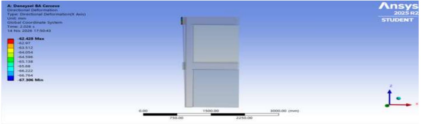
Şekil 6.2 Referans Numune x Yönünde Çerçeve 2. Kat Tepe Deplasmanı
