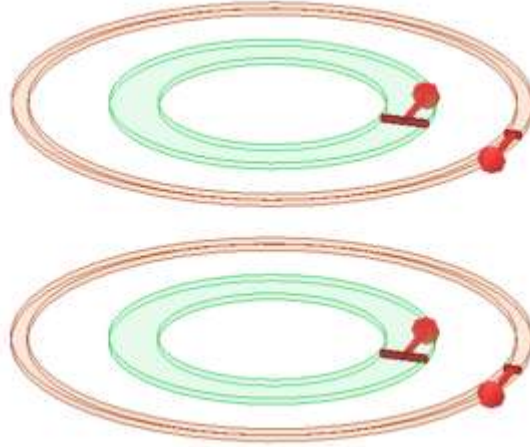
Şekil 4. Aktif ekranlama bobini kullanan bir EAG’ın 3D görüntüsü
