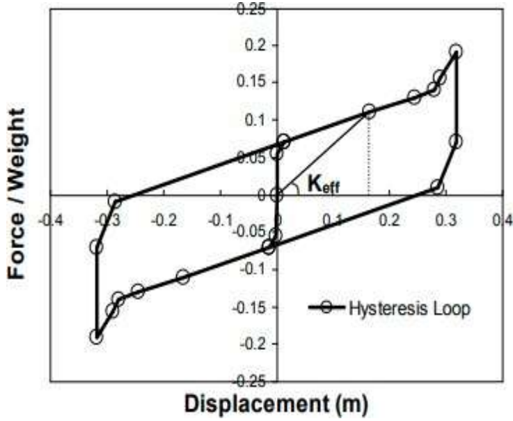
Şekil 2.1 İdealleştirilmiş doğrusal olmayan histerezis modeli üçlü sürtümlü sarkaç izolatörü için eğri [66]
