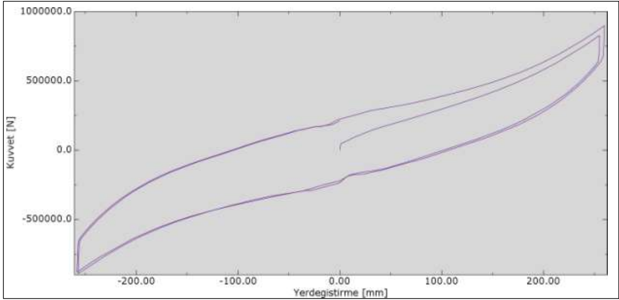
Şekil 3.4 Kurşun çekirdekli kauçuk izolatör
