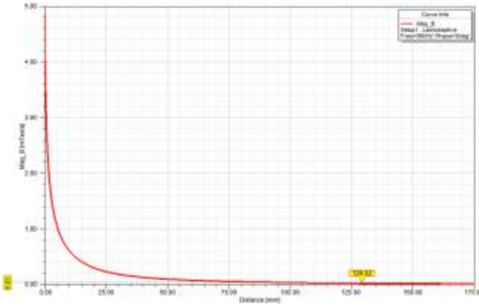
Primer sargı hizasında akı yoğunluğu değişimi
