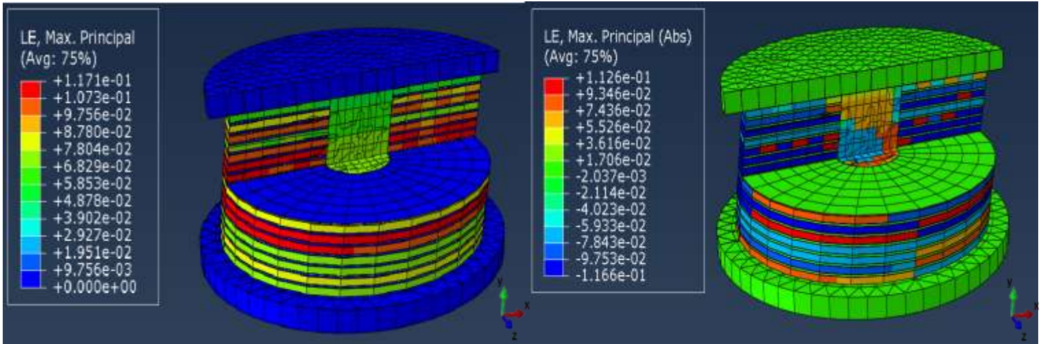
Şekil 3.1 Kurşun Çekirdekli Kauçuk İzolatörün Logaritmik Deformasyonu
