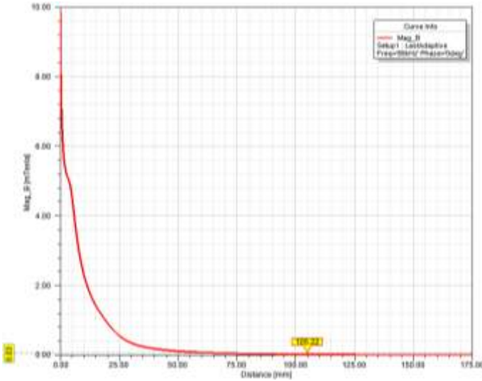
Şekil 5. Ekranlama modellerinin incelenen düzlemler boyunca manyetik akı yoğunluğu değişimleri
