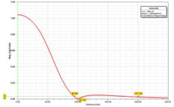
Orta yükseklik hizasında akı yoğunluğu değişimi
