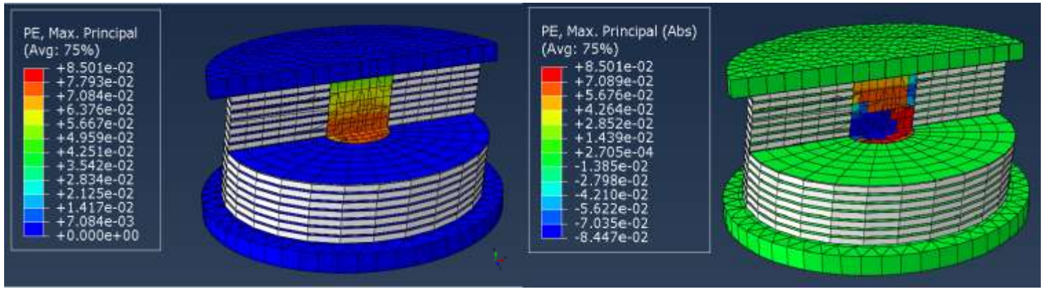
Şekil 3.1 Kurşun Çekirdekli Kauçuk İzolatörün Plastik Deformasyonu
