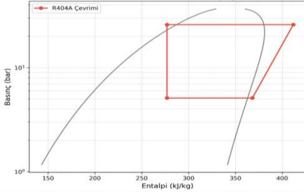
Şekil 2. Tasarlanan Sistem: R290 Akışkanının +55°C Yoğuşma Şartlarındaki P-h diyagramı
