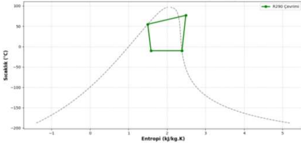
Şekil 5. Tasarlanan sistem R290 T-s diyagramı
