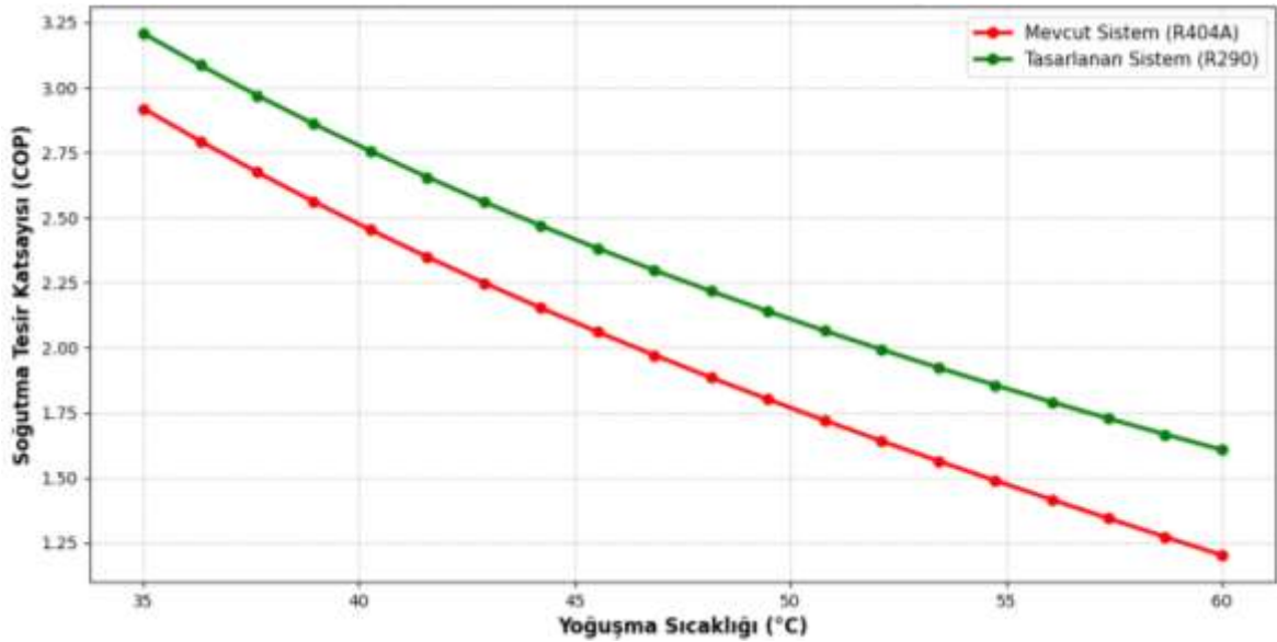
Şekil 6. Dış ortam yoğuşma sıcaklığına bağlı olarak sistemlerin COP değişimi
