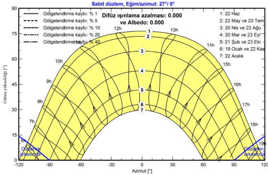
Şekil 2. Şanlıurfa bölgesinde yıl içindeki güneş yörüngesi
