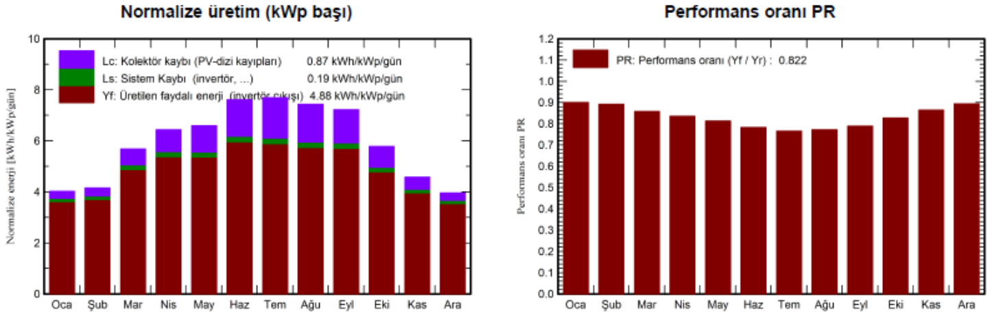
Şekil 3. Şanlıurfa bölgesindeki panelin yıllık enerji üretimi ve performans oranı
