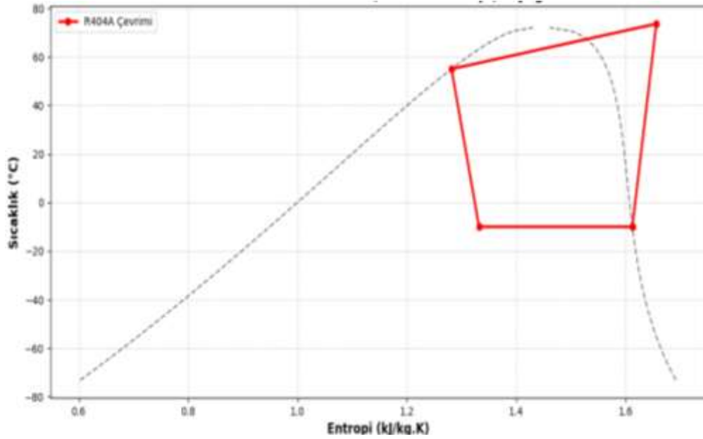
Şekil 4. Mevcut sistem: R404A T-s diyagramı
