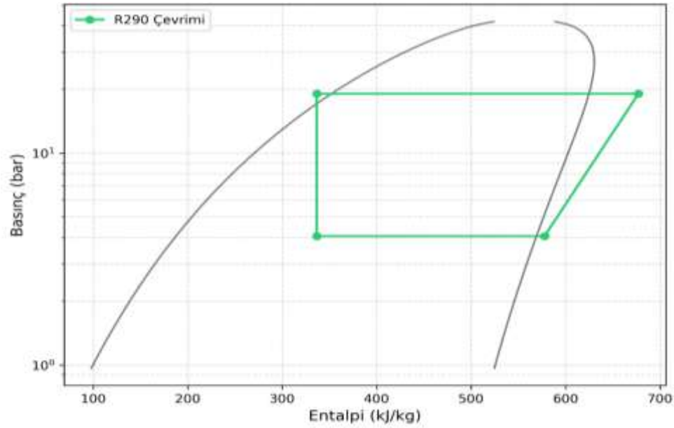
Şekil 3. Tasarlanan sistem: R290 akışkanının +55°C yoğuşma şartlarındaki P-h diyagramı
