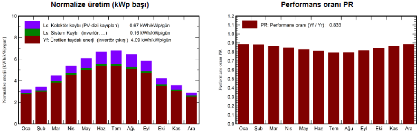
Şekil 4. Antalya bölgesindeki panelin yıllık enerji üretimi ve performans oranı
